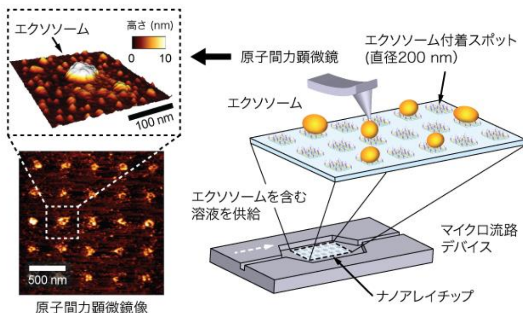
図1 本研究で開発した、エクソソームを平面配列化するナノアレイプラットフォーム ナノアレイチップ表面には、脂質分子が修飾された付着スポットが高密度に形成されています。マイクロ流路デバイスにナノアレイチップを取り付けて、エクソソームを含む溶液を流すと、スポット上にエクソソームが付着します。デバイスからナノアレイチップを取り出せば、原子間力顕微鏡などを用いて、エクソソームの個別解析が可能です。
